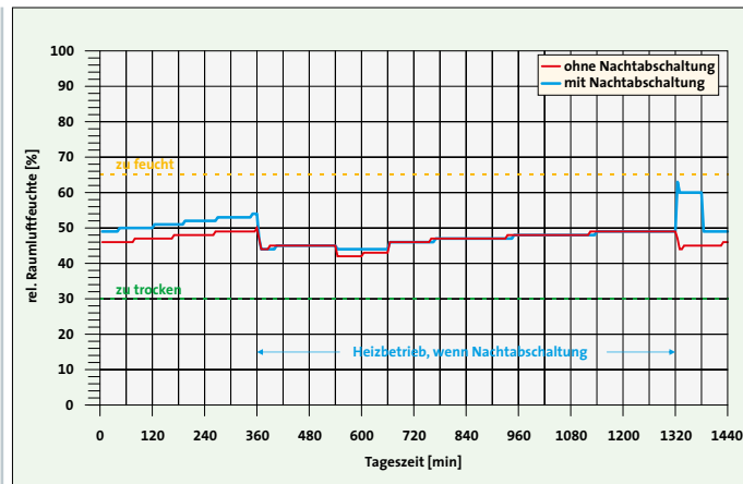
Bild 2a: Feuchte-Simulation mit dem C.A.T.S.-Kühllastprogramm (Rahmenbedingungen: Schlafzimmer in Wohnung nach EnEV 2007 gebaut mit 2 x 10 min Stoßlüftung am Tag (2 Personen, 2 Topfpflanzen, Wäschetrocknen, Feuchteproduktion: 888 g/Tag))
